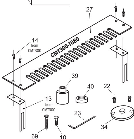
Mini incastri a denti diritti (CMT300-T080)
