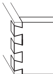
Encajes de cola de milano abierta ( CMT300-T129 )
