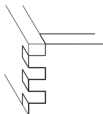
Mini-encastresments à dents droites (CMT300-T080)
