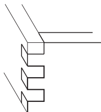
Mini incastri a denti diritti (CMT300-T080)
